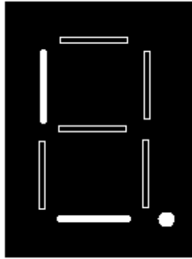
รูปที่ 2-2 แสดงการติดของ LED เมื่อเข้าสู่โหมดการโหลดข้อมูล
