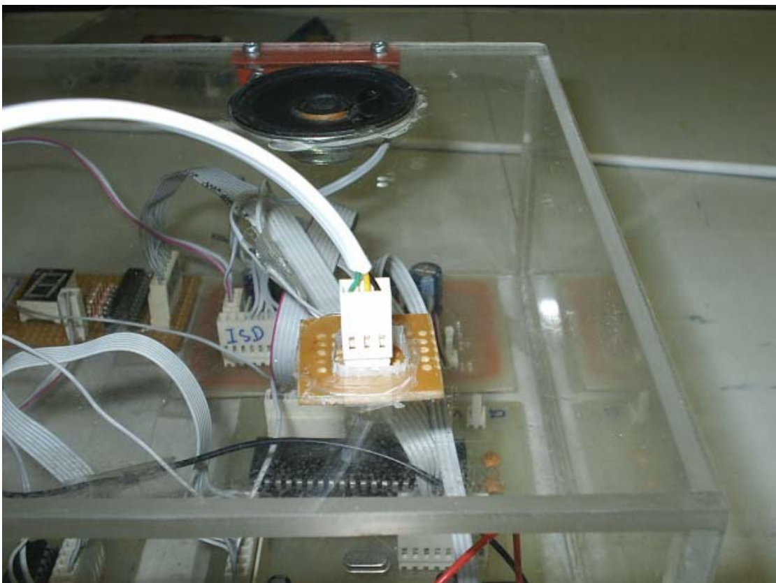
รูปที่ 2-1 แสดงการต่อสายลิงค์เข้ากับคอนเน็คเตอร์
