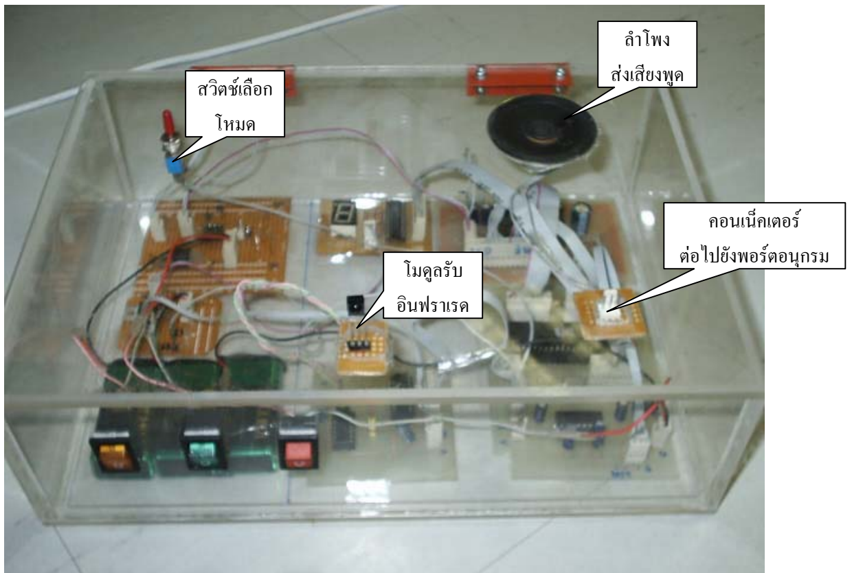
รูปที่ 1-3 แสดงเครื่องรับเมื่อมองจากด้านบน
