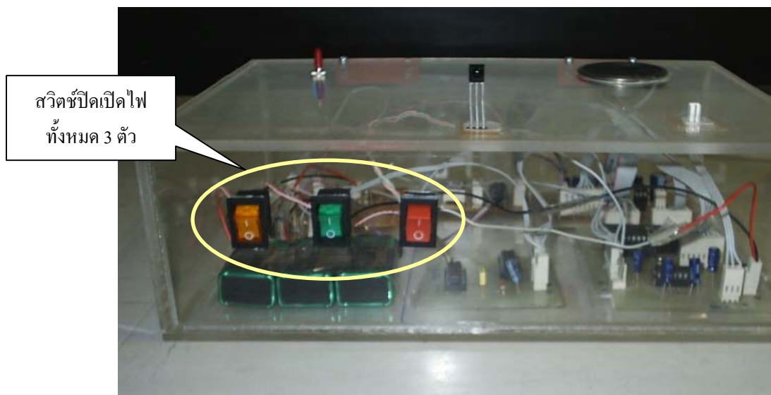
รูปที่ 1-2 แสดงเครื่องรับเมื่อมองจากด้านหน้า
