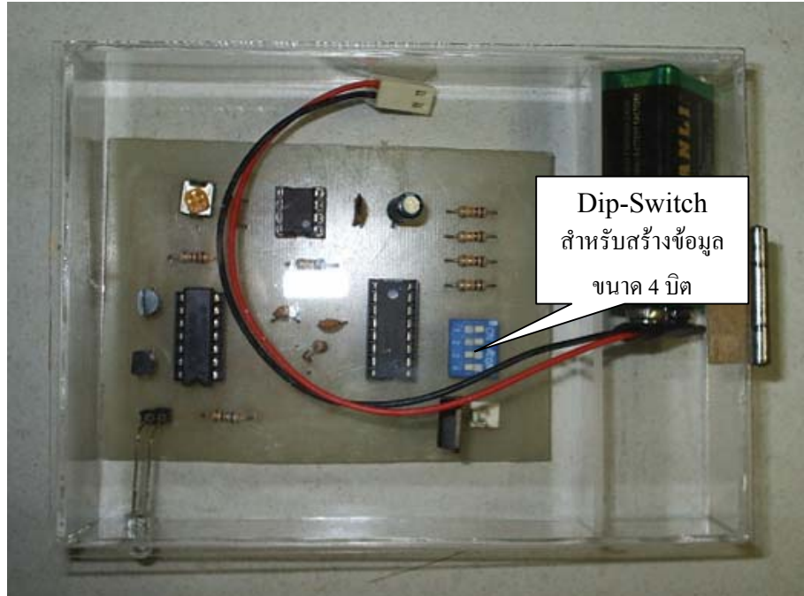
รูปที่ 1-1 แสดงเครื่องส่ง
